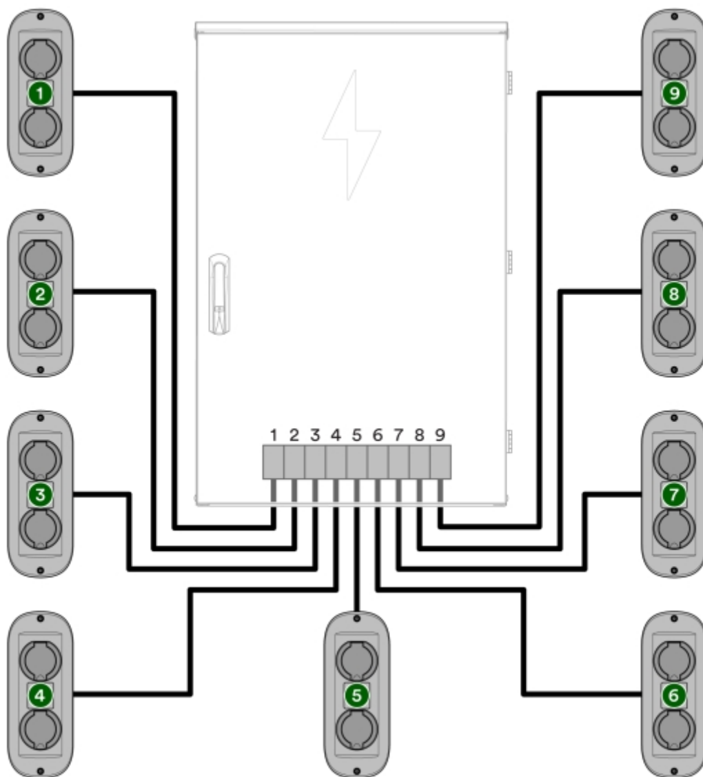
Bild 31: Adressering 9 switchar
