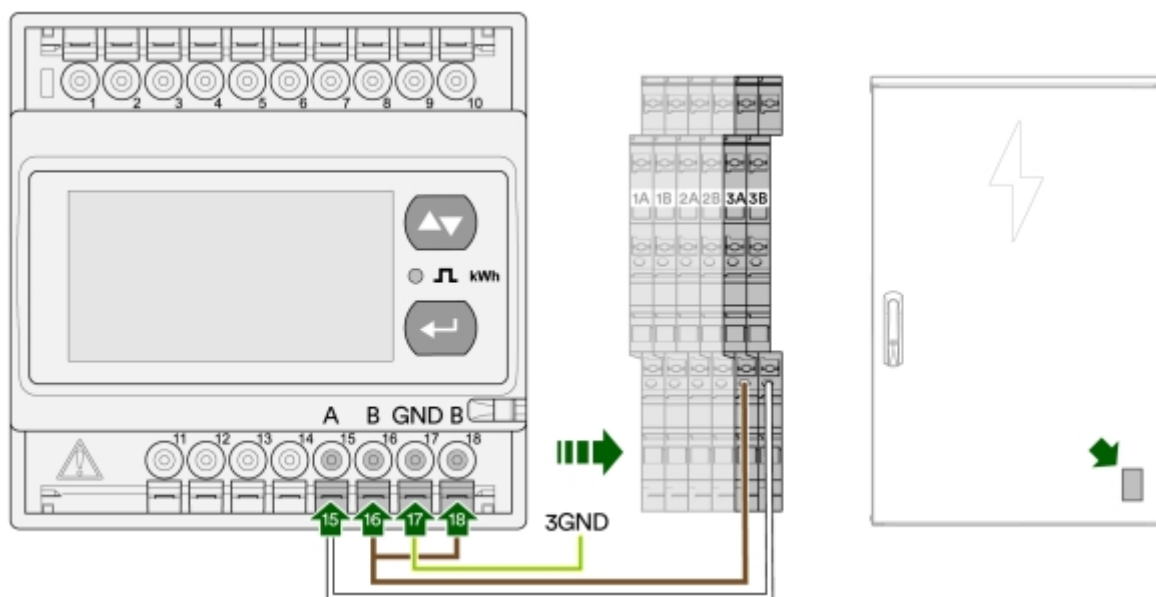
Bild 53: Ingångar 15-18 på energimätaren
