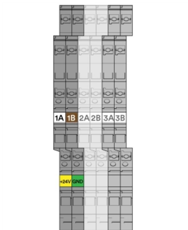
Bild 23: Inkoppling till laddcentral
