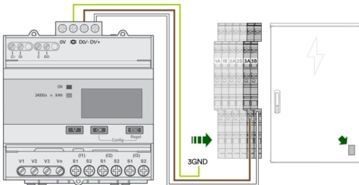
Bild 58: Ingångar för RS485
