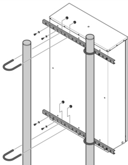
Bild 8: Montering av laddcentral på stolpar
