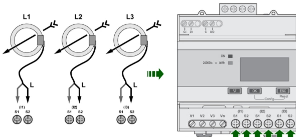
Bild 56: Ingångar för strömtransformator
