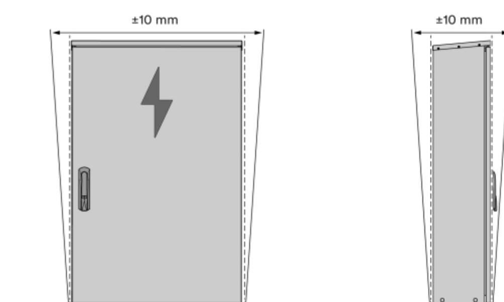
Bild 7: Kontroll av rakhet
