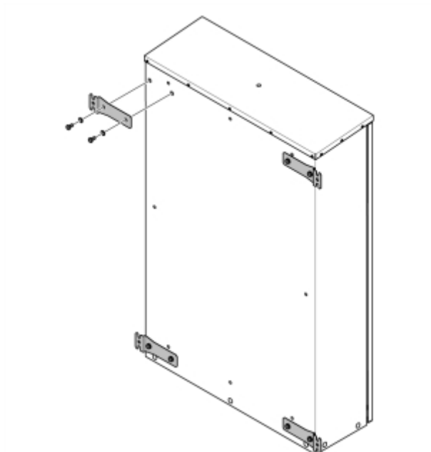
Bild 6: Väggfästen på laddcentral
